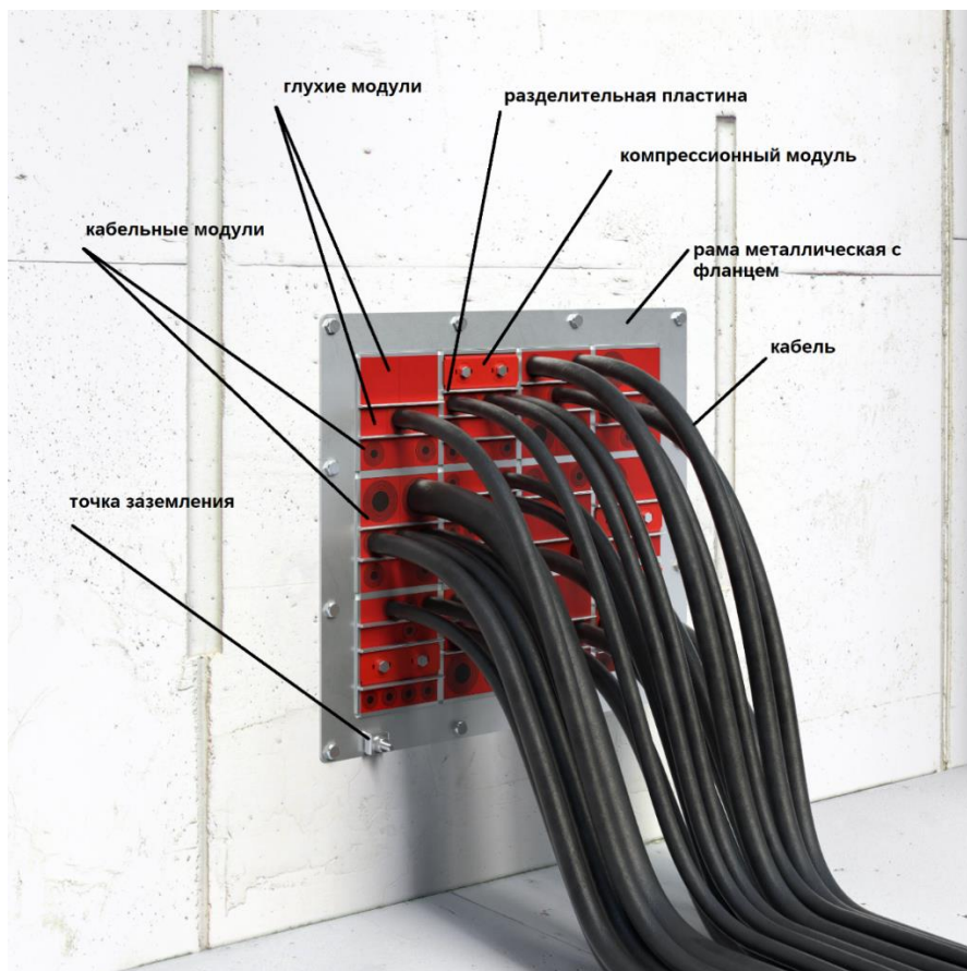
Рисунок 1 – Кабельная проходка на основе металлической рамы с фланцем
